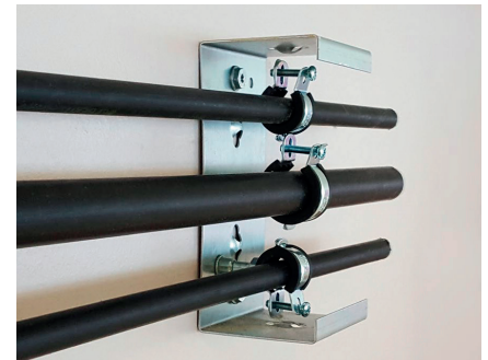
Putket ja kotelot seinään samoilla kannakkeilla. Kuvassa 80 x 180 mm kannake.
