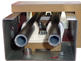
Putket ja kannakkeet L-kotelossa (60x100 mm)
